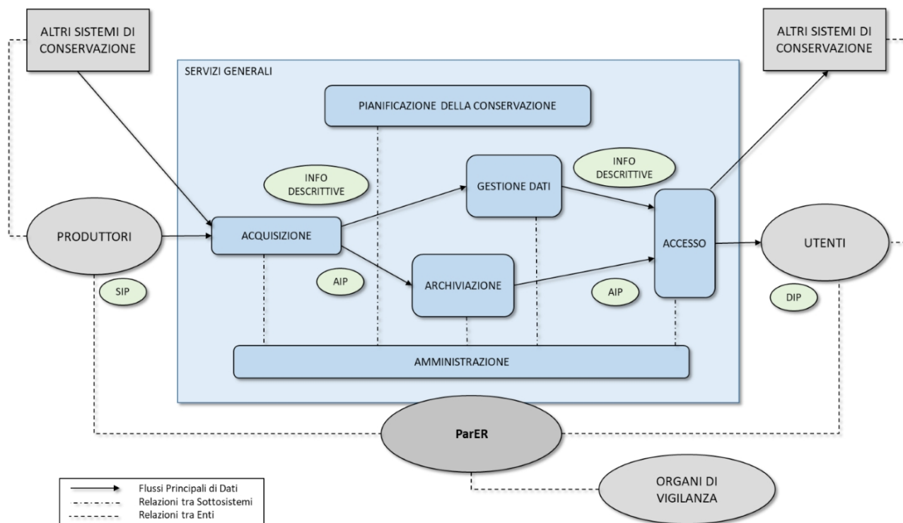
Figura 1 Schema logico del Sistema di conservazione dal Manuale ParER
